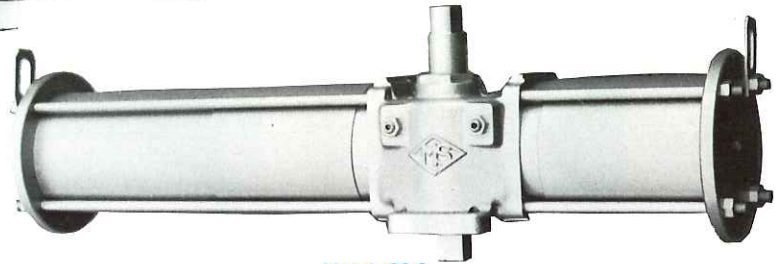
Model CS-2 单动式传动器 Actuator (Torque 550~1260 kg·cm)
