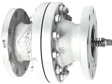
Model EFV-F 法兰盘形 过量排流阀(¼"~14") Flanged Excess Flow valve
